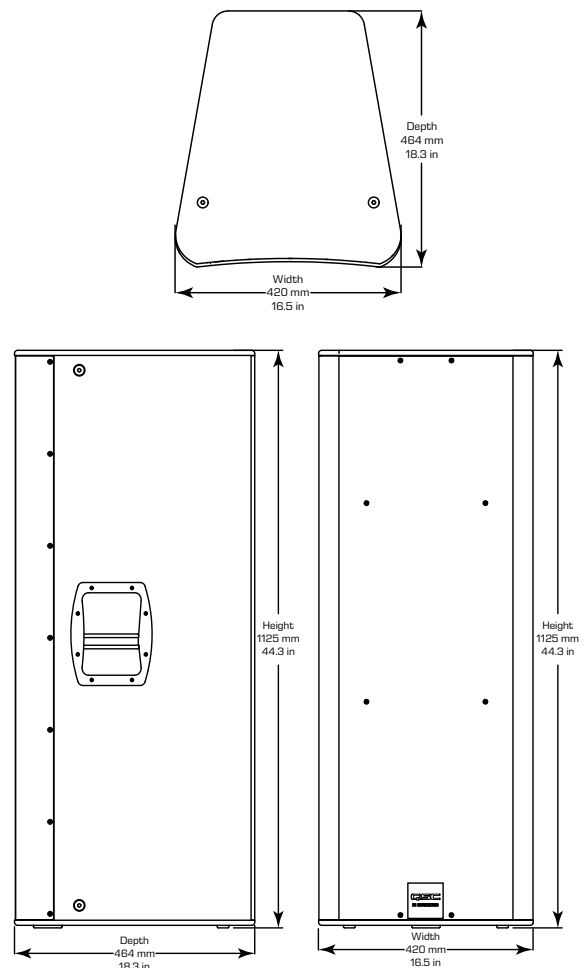
E215 Dimensions
